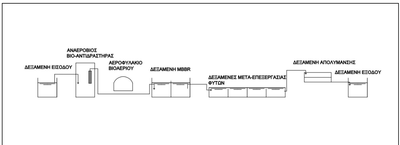
Εικόνα 1. Διάγραμμα ροής πιλοτικής μονάδας
