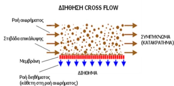
Σχήμα: Σχηματική απεικόνιση της διήθησης τύπου cross flow
