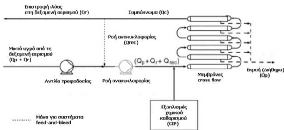
Σχήμα: Τυπικό διάγραμμα ροής συστήματος με εξωτερικές μεμβράνες τύπου cross-flow για διαχωρισμό βιομάζας σε βιοαντιδραστήρα μεμβρανών
